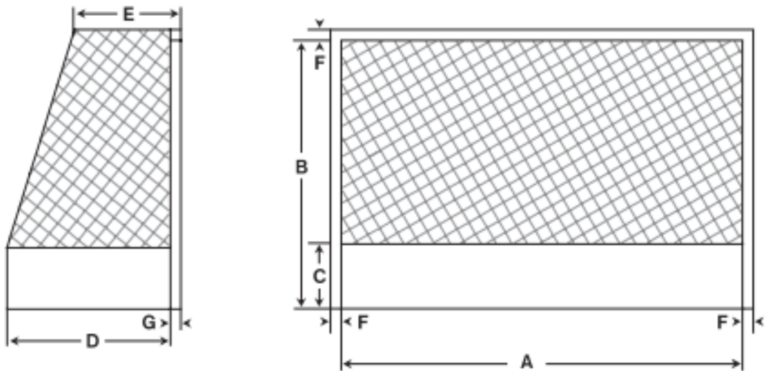
Dimensiones del arco
