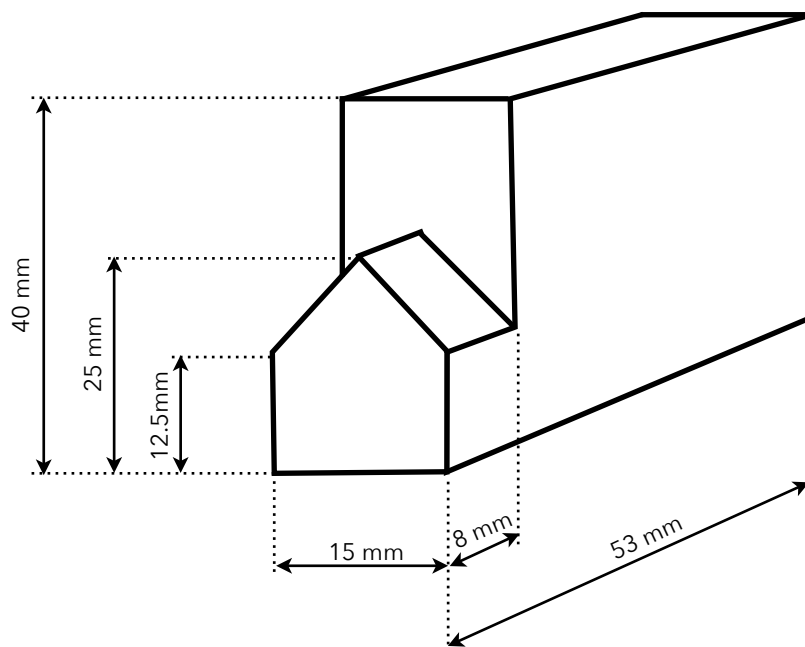
Figura 6: Dispositivo para medir el arco o inclinación del palo
